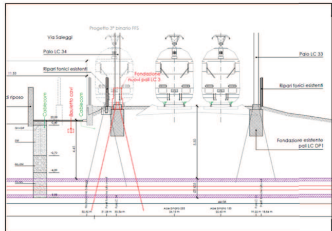
Sezione asse spingitubo
